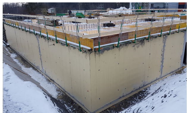
Fouille à ciel ouvert avec SikaProof® A+ : après dépose des coffrages, les trous de banche doivent être étanchés.
